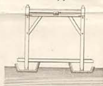
Przecięcie poprzeczne.
